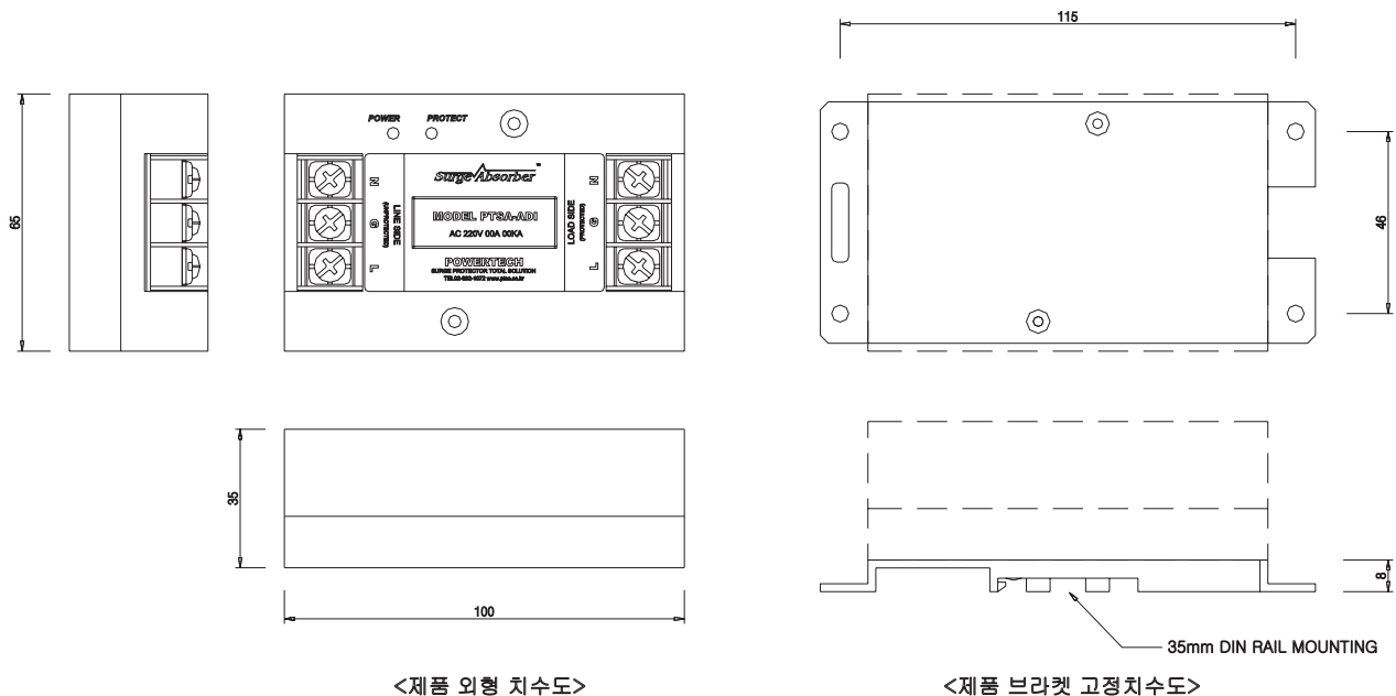
<제품 외형 치수도>
